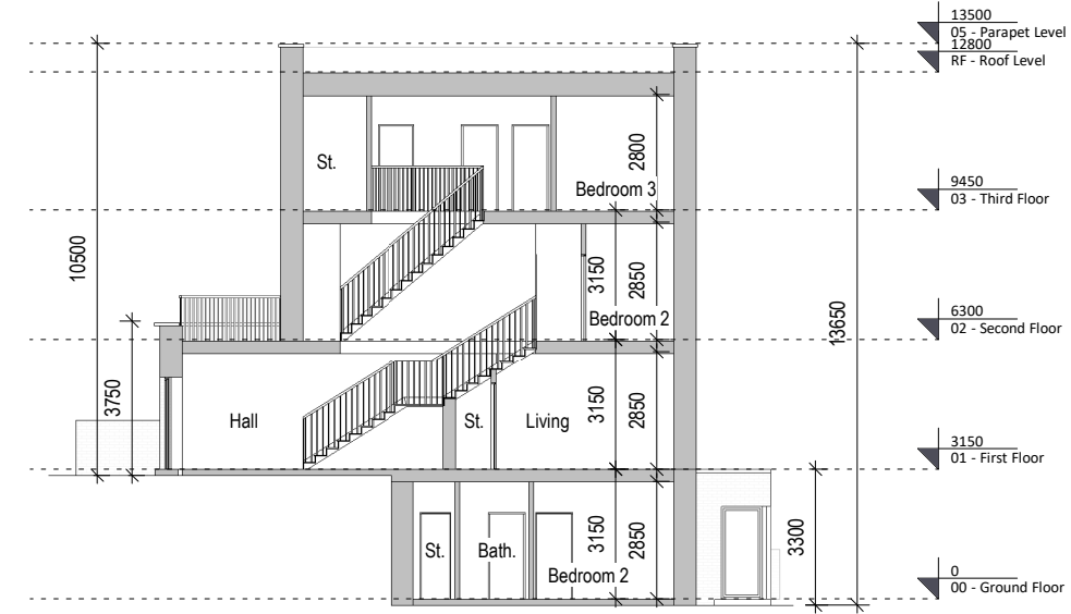
4 Section 1 1 : 200
