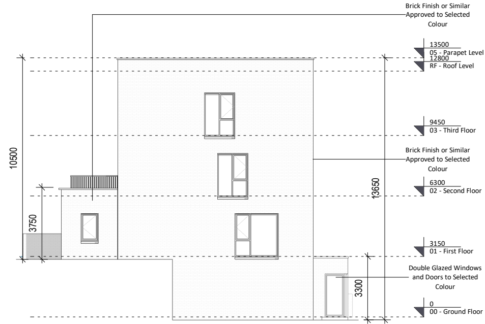
2 Left Elevation 1 : 200
